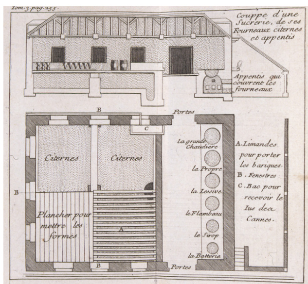
Coupe d'une Sucrerie, de ses Fourneaux citernes et apprentis. Gravure extraite de l'ouvrage « Nouveau voyage aux isles de l'Amérique », du père Jean-Baptiste Labat.
