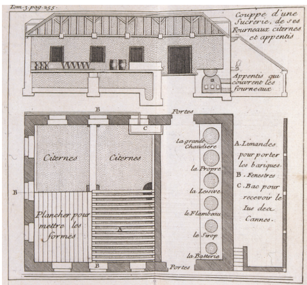
Coupe d'une Sucrierie, de ses Fourneaux citernes et apprentis. Gravure extraite de l'ouvrage « Nouveau voyage aux isles de l'Amérique », du père Jean-Baptiste Labat.
